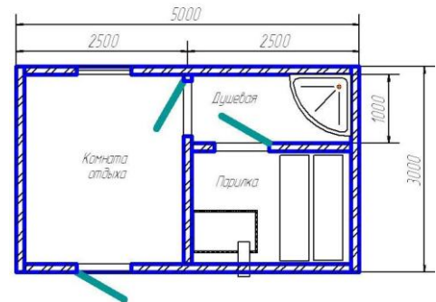
БСММ 3,0x5,0x2,5м
