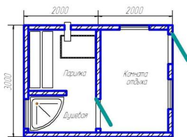
БСММ 3,0x4,0x2,5м
