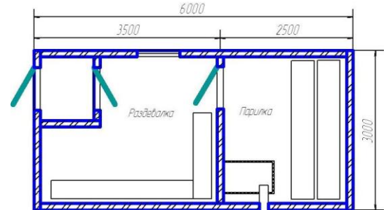
БСММ 3,0x6,0x2,5м
