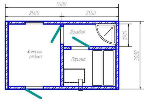
БСММ 3,0x5,0x2,5м
