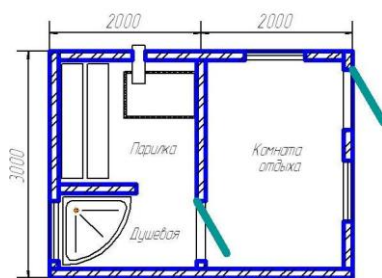
БСММ 3,0x4,0x2,5м
