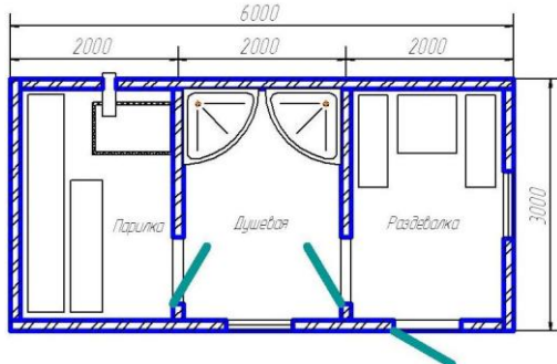
БСММ 3,0x6,0x2,5м
