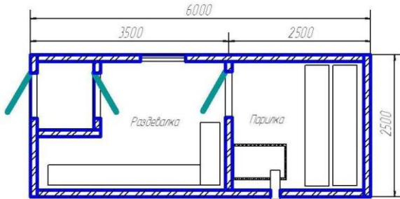
БСММ 2,5x6,0x2,5м
