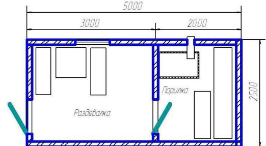
БСММ 2,5x5,0x2,5м
