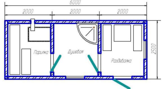
БСММ 2,5x6,0x2,5м
