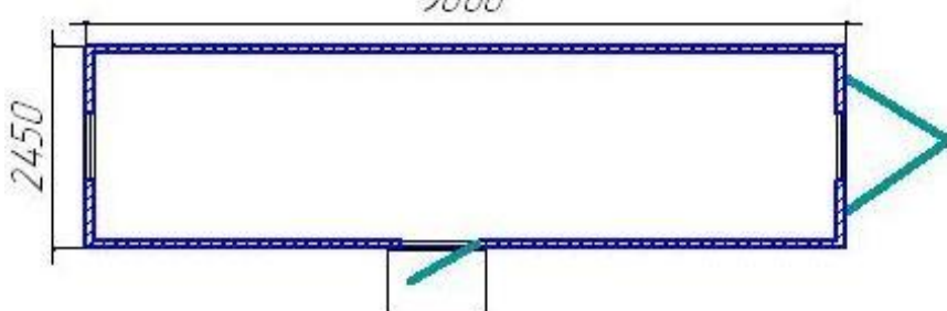
Вагон-дом на шасси (ВДШ)
