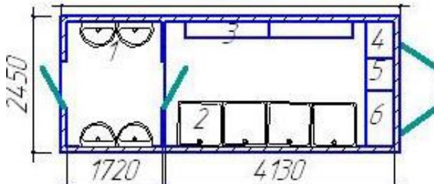
Вагон-дом душевая (ВДШд)
