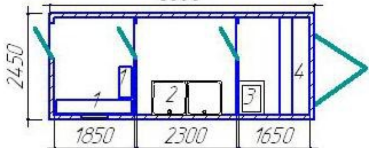
Вагон-дом баня-сауна (ВДШбс)
