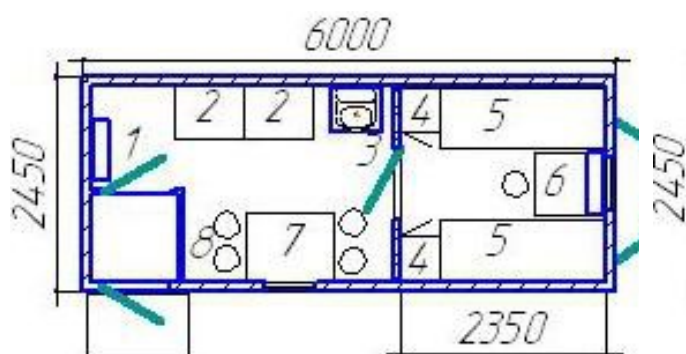
Вагон-дом жилой (ВДШж) на 4 чел. 2,5x6,0-2,5 (3,8)м
