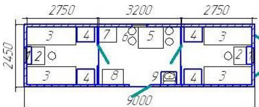
Вагон-дом жилой (ВДШж) на 8 чел. 2,5x9,0-2,5 (3,8)м
